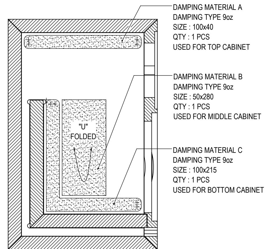
SECTION A-A SCALE 2 : 5
